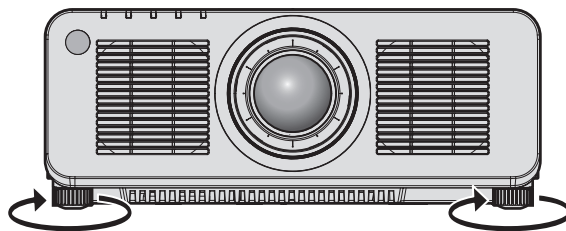
최대 조절 가능 범위 조절식 발: 각각 30 mm (1-3/16")
