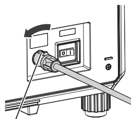
잠금 레버
